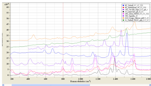
7. kép – Kék színű golyósíron színezőpaszták Raman spektrumai (URL1)
